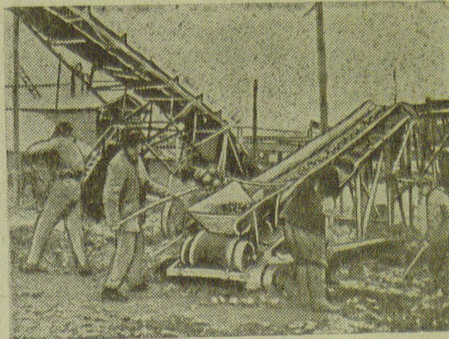
На головном сооружении. На снимке: транспортер в работе.
